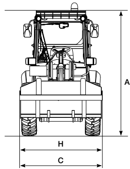
Pala gommata con benna standard e pneumatici standard (vista frontale)
