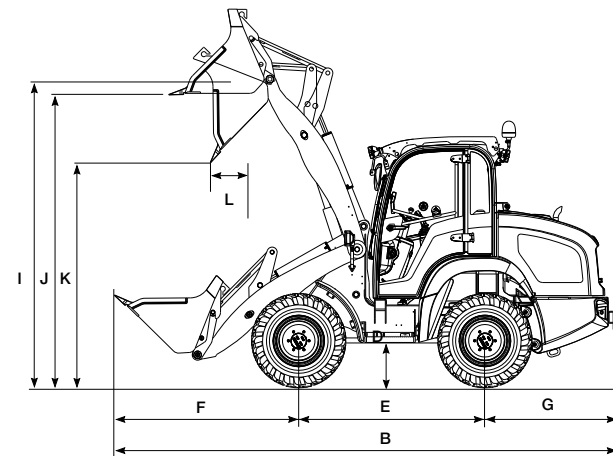
Pala gommata con benna standard e pneumatici standard (vista laterale)
