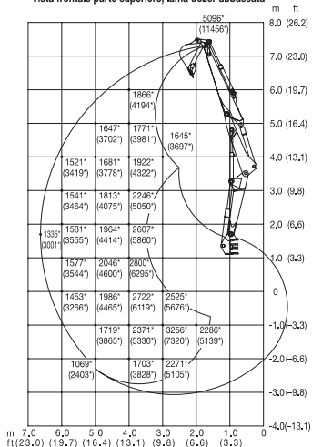
Vista frontale parte superiore; lama dozer abbassata
