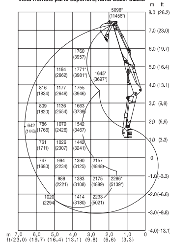
Vista frontale parte superiore; lama dozer alzata
