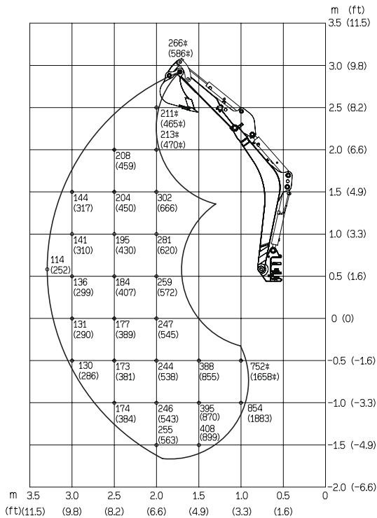
Vista frontale parte superiore; lama dozer alzata
