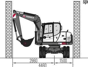
Fig. 2: Cerchio tangente
